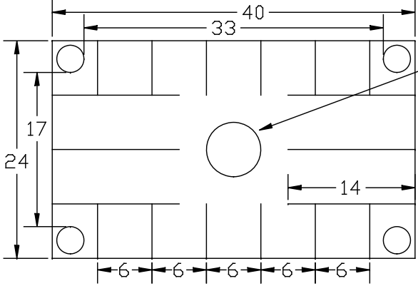
BED PLATEN LAYOUT
