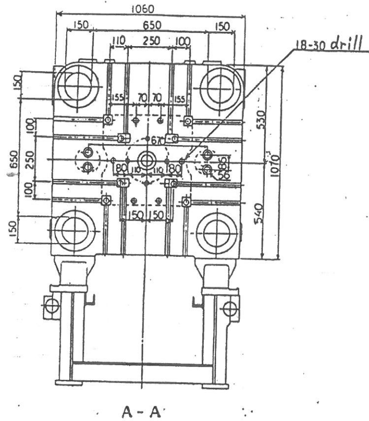
Moving platen
